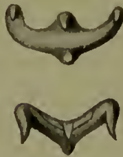
Fig. 150. Chitinhaken vom Kopf des Triaen. nodulosus (nach Wagener).
